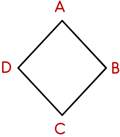
ABCD dörtgeni
